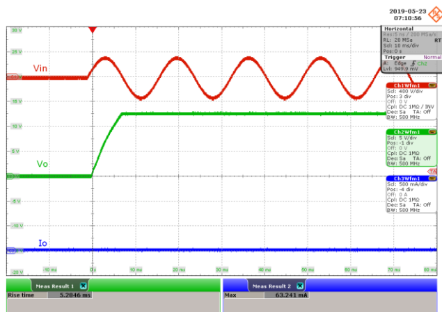
CH1: V_{IN} , 400 V / div., 10 ms / div. CH2: V_{OUT} , 5 V / div., 10 ms / div. CH3: I_{OUT} , 500 mA / div., 10 ms / div. Rise Time = 5.2846 ms.
