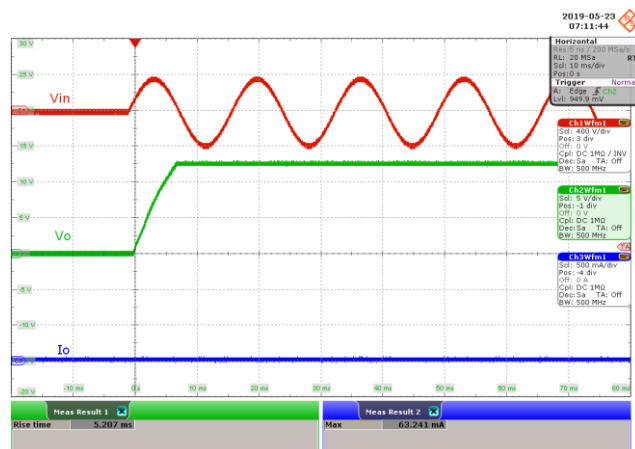
CH1: V_{IN} , 400 V / div., 10 ms / div. CH2: V_{OUT} , 5 V / div., 10 ms / div. CH3: I_{OUT} , 500 mA / div., 10 ms / div. Rise Time = 5.207 ms.
