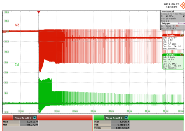
Figure 69 – 230 VAC 50 Hz. CH1: V_D , 20 V / div., 10 ms / div. CH2: I_D , 2 A / div., 10 ms / div. PIV = 78.972 V, I_{D(MAX)} = 4.996 A.
