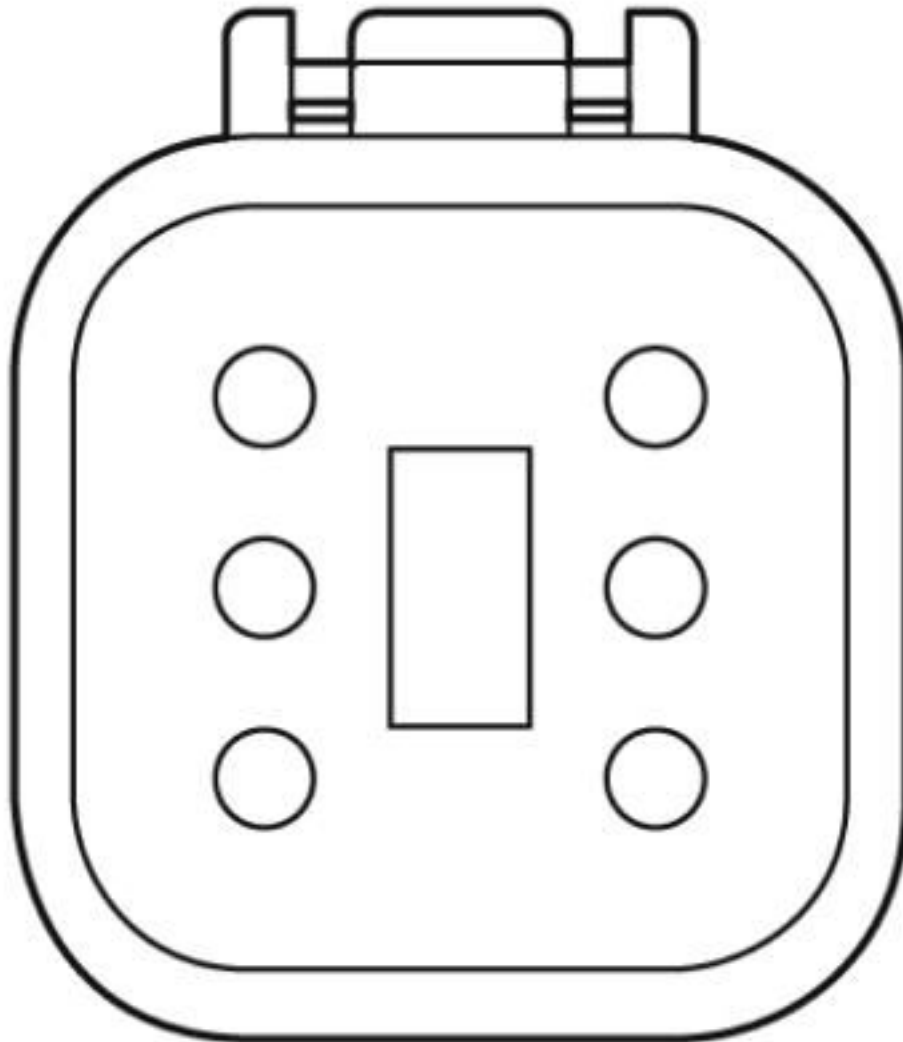
DEUTSCH DT06-6S pin assignment
