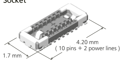
Socket
