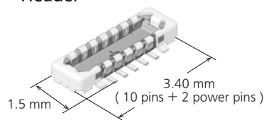
Header
