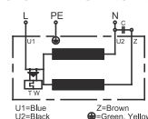
MOTOR WIRING DIAGRAMS
