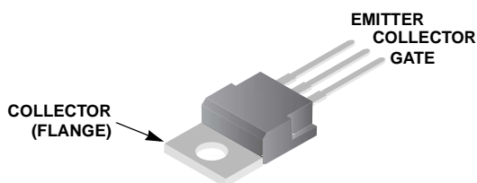
JEDEC TO-220AB
