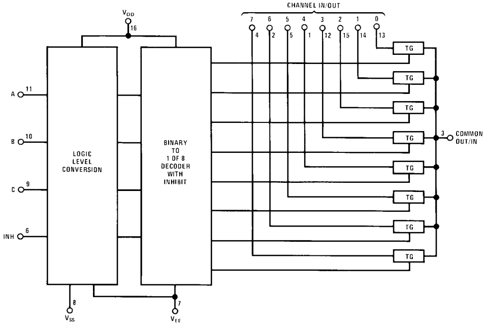
CD4051BC
