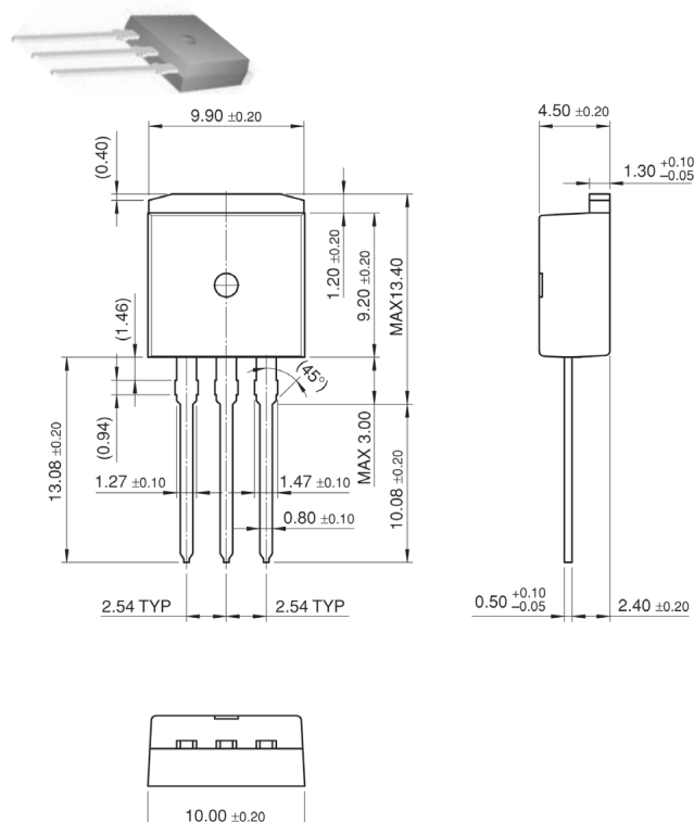
TO-262 (I 2 PAK)
