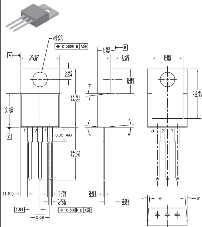
TO-220/TO-220AB
