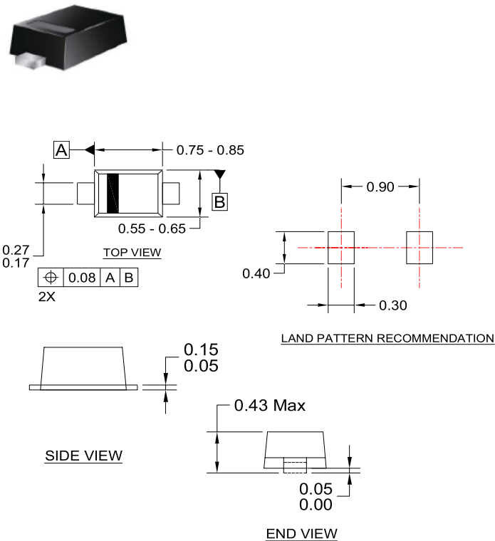
SOD-923
