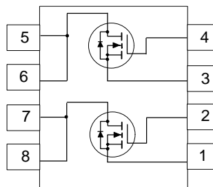
SO-8
