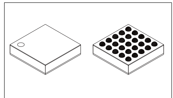
WLP25J(2.17X2.17)
