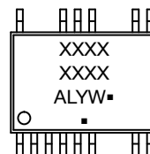
TSSOP20 CASE 948BL
