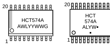
SOIC-20
