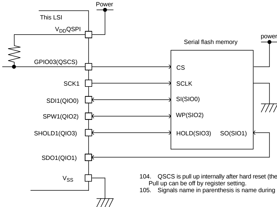
Figure 49. S-Flash I/F
