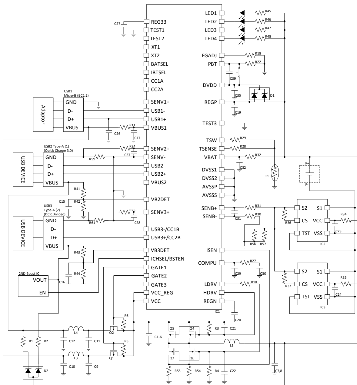
USB Type-C VBUS CC1 CC2 GND LC709511F VBUS1 CC1A CC2A SENV1+ SENV- C40 C41 R58 IC1
