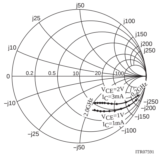
S22e f=200MHz to 2000MHz(200MHz Step)
