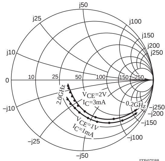
S11e f=200MHz to 2000MHz(200MHz Step)
