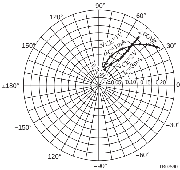
S12e f=200MHz to 2000MHz(200MHz Step)
