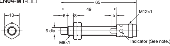
E2A-S08LN04-M1-□□ E2A-M08LN04-M1-□□
