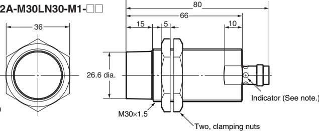
E2A-M30LN30-M1-□□
