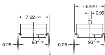
Flat Actuator
