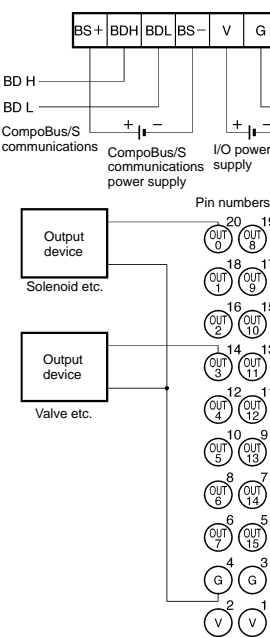
SRT2-VOD16ML-1
