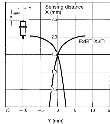
E2E2-X□C□/B□
