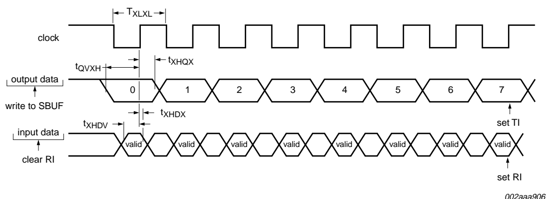
Fig 24. Shift register mode timing
