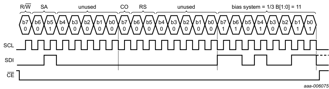
Fig 45. SPI-bus example
