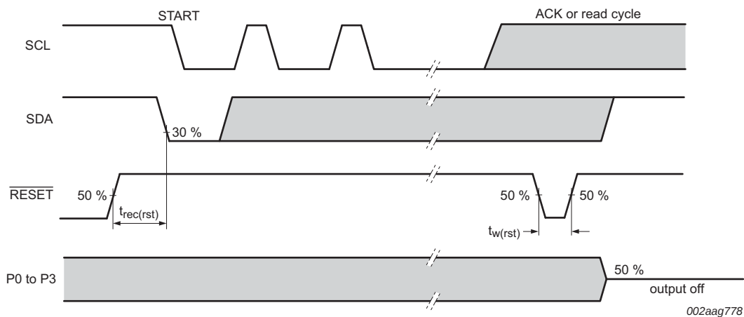
Fig 27. Reset timing
