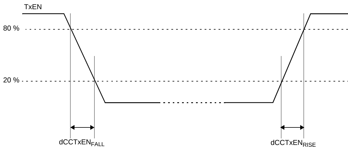
Figure 46. TxEN signal
