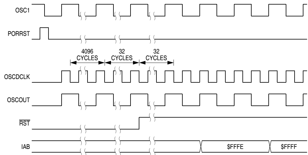
Figure 8-7. POR Recovery
