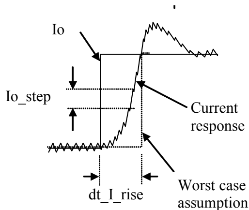
Figure 8. Transient Parameters
