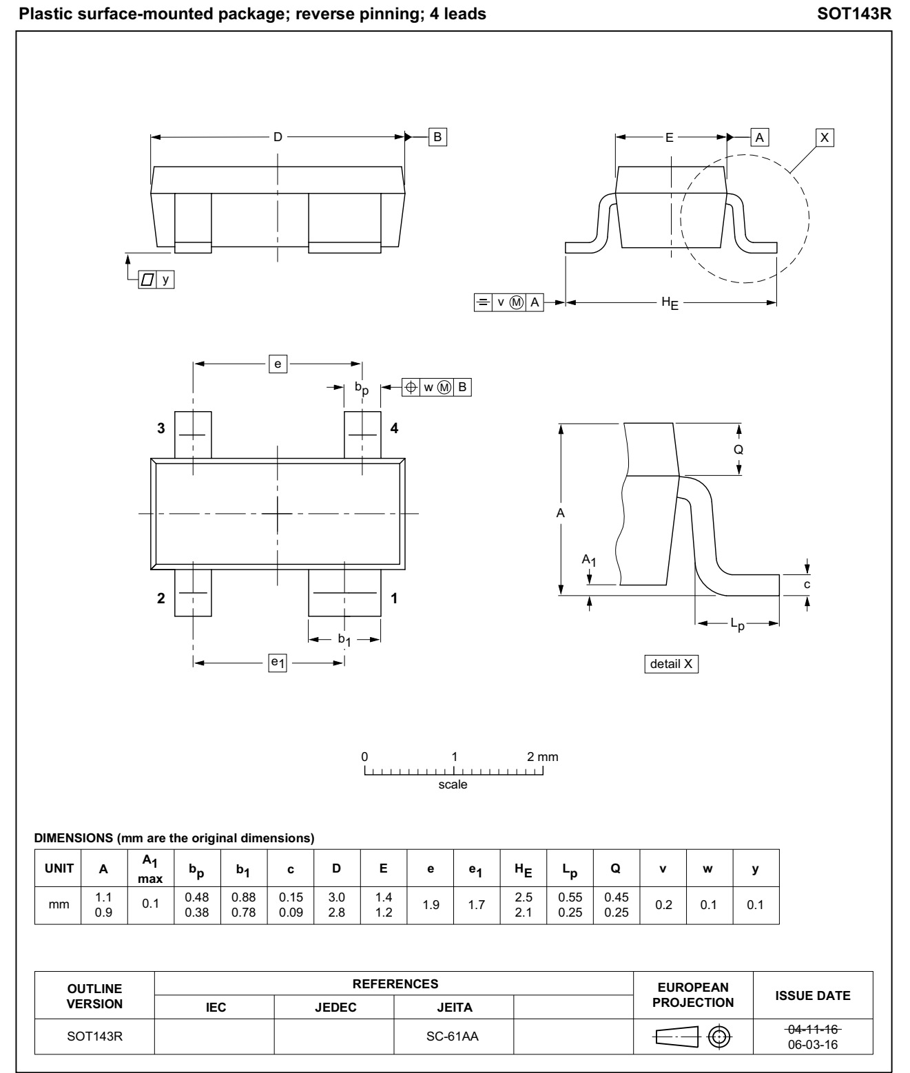
Fig 27. Package outline SOT143R
