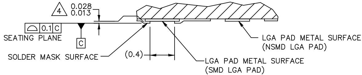
SECTION E-E △ 5
