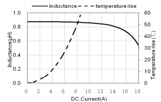
ASPIAIG-S8050-1R0
