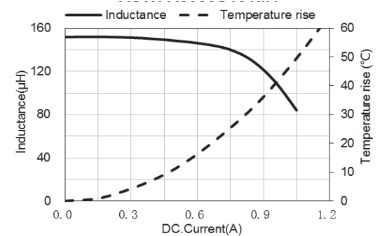
ASPIAIG-S6055-151
