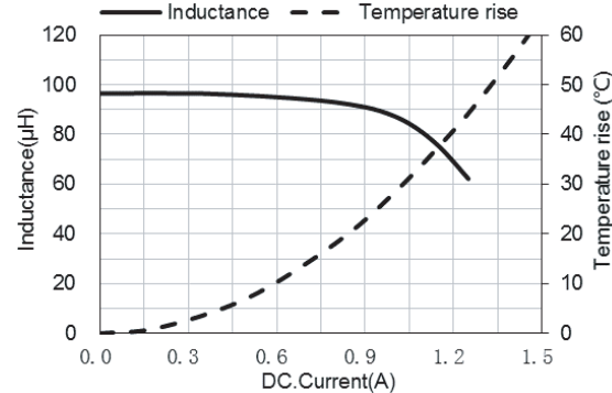
ASPIAIG-S6055-101
