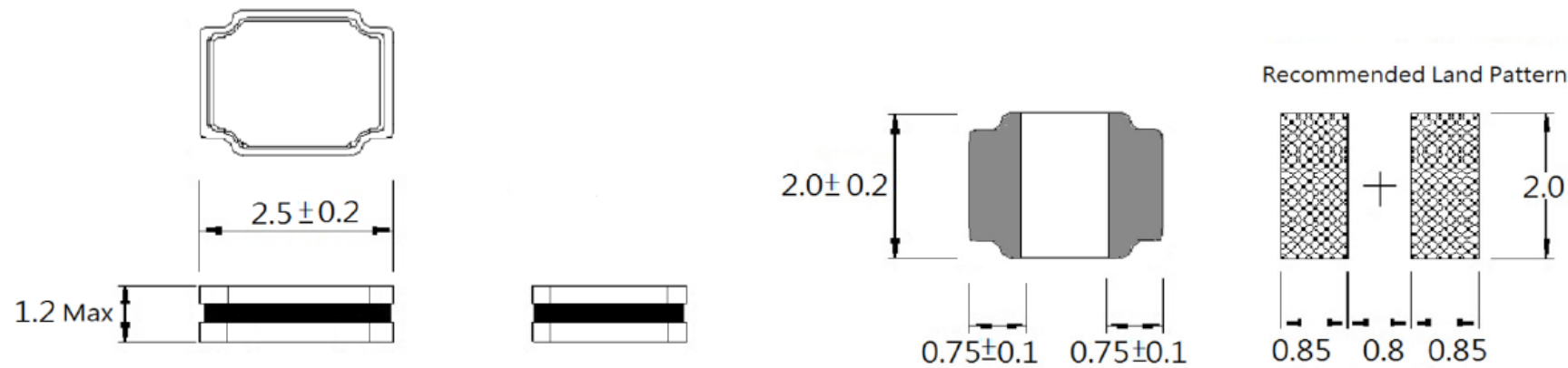
ASPI-M2512
