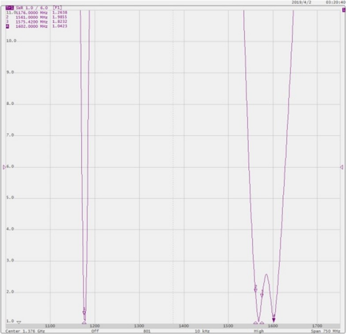
VSWR
