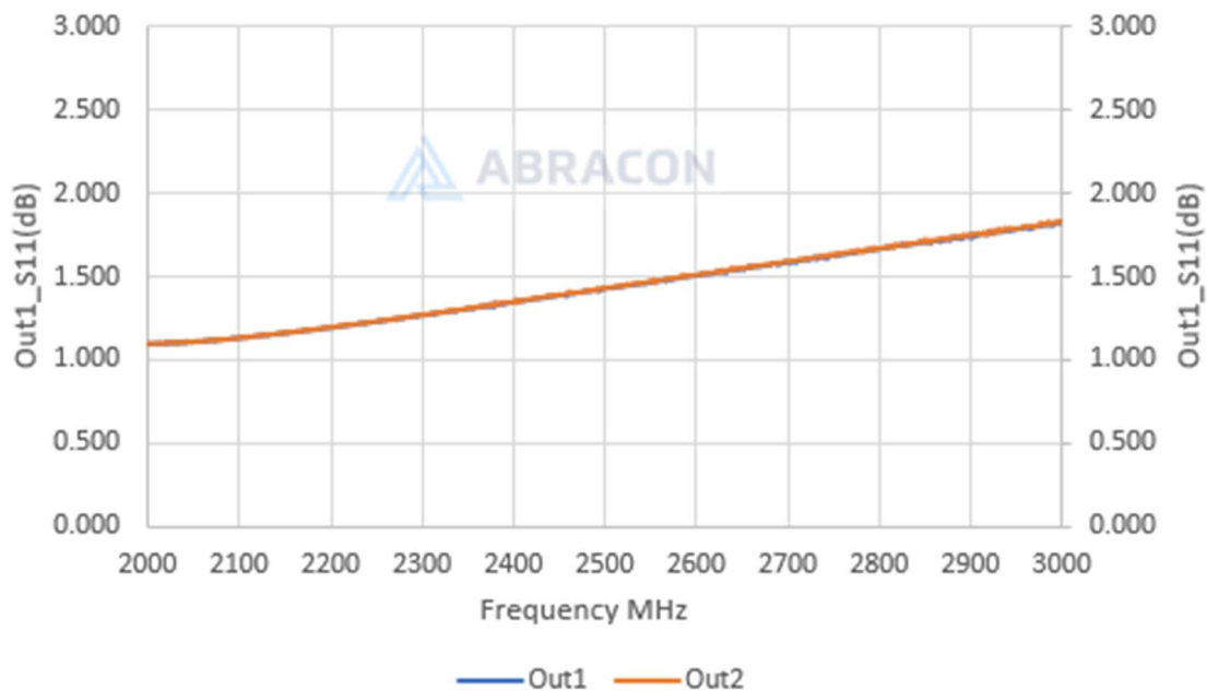
VSWR_S11(2300-2700MHz)
