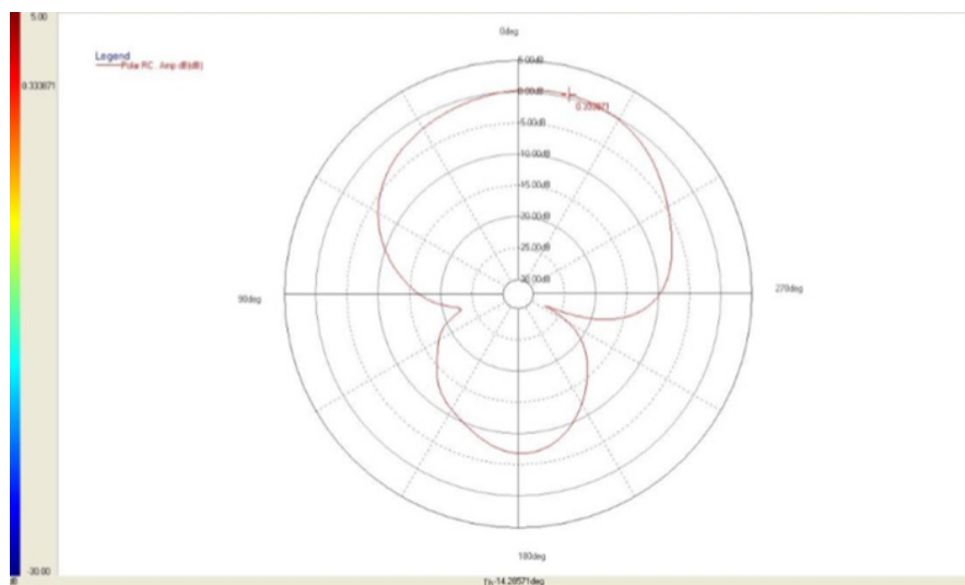
YZ-Plane 1227 MHz
