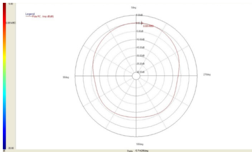
XZ-Plane 1227 MHz
