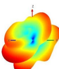
LTE 1710 MHz
