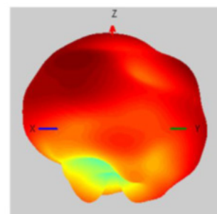
1850MHz
