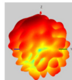
5800MHz
