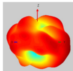
2690MHz
