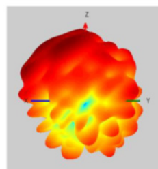
5925MHz
