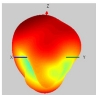
960MHz
