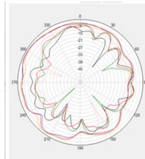
YZ-PLANE
