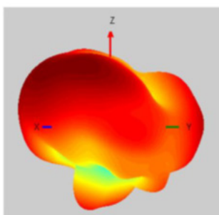
1710MHz
