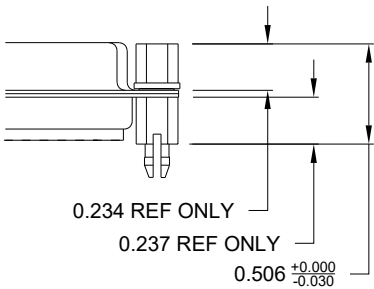
"91" // PCB SIDE
