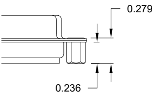
"02" // PCB SIDE
