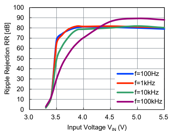
NR1640DC330x, I_{OUT} = 100\text{ mA}
