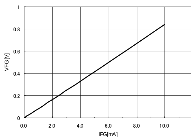
VFG-IFG VDD=12V
