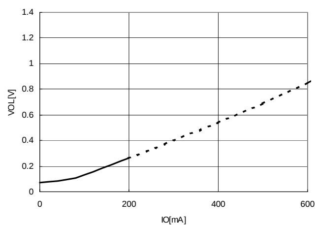
IO-VOL VDD=12V
