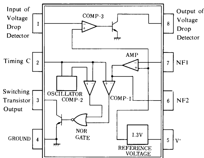
NJM2352D NJM2352M
