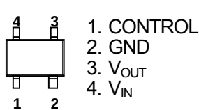
NJM2878F4
