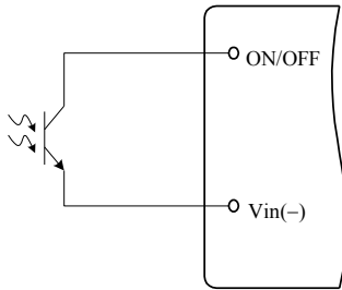
Fig. 13 Opto Coupler Enable Circuit
