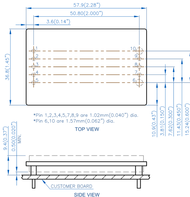
Open Frame Module
