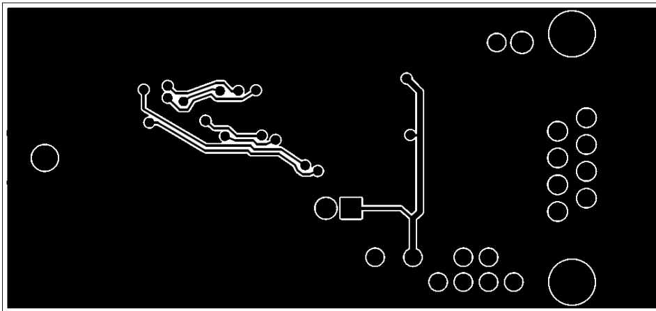
Bottom Side
