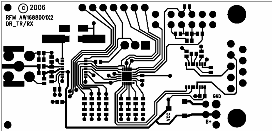
Top Side
