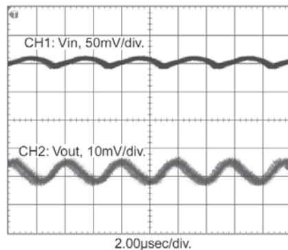
7812SR-C V_{IN} = 24\text{V} , I_{LOAD} = 40\text{mA}
