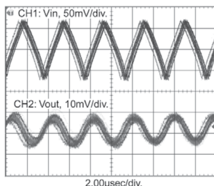
7812SR-C V_{IN} = 24\text{V} , I_{LOAD} = 400\text{mA}
