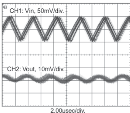
7805SR-C V_{IN} = 12\text{V} , I_{LOAD} = 500\text{mA}
