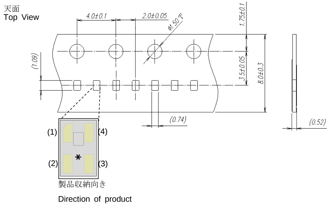
第2図 プラスチックテープの外形寸法図
