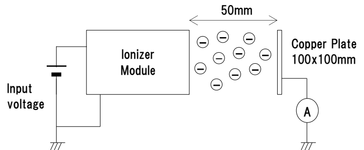
《 図 1-b 》イオン測定方法(微小電流計)
