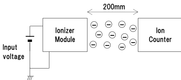
《 図 1-a 》イオン測定方法(イオンカウンター)
