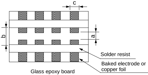
Fig.3 (in:mm)
