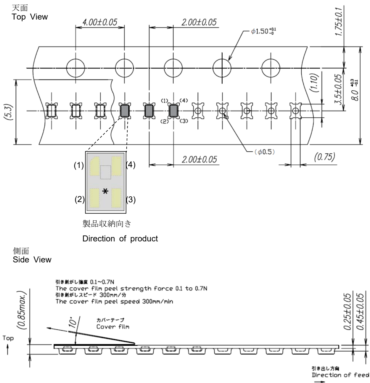
第2図 プラスチックテープの外形寸法図
