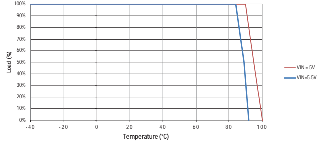
MGJ2D121505MPC
