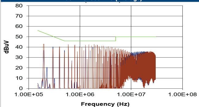
MGJ2D152005MPC (Average)
