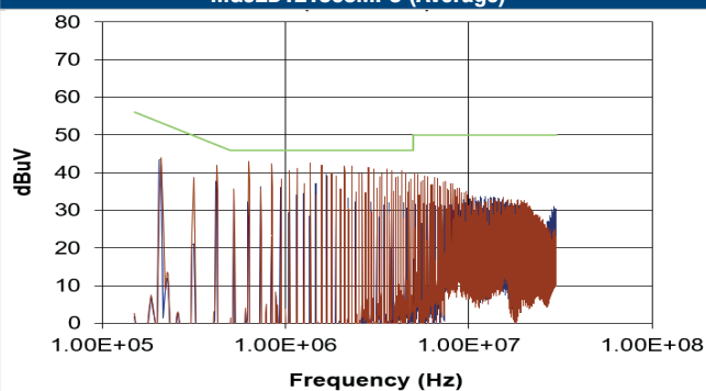
MGJ2D121509MPC (Average)
