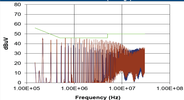
MGJ2D122005MPC (Average)
