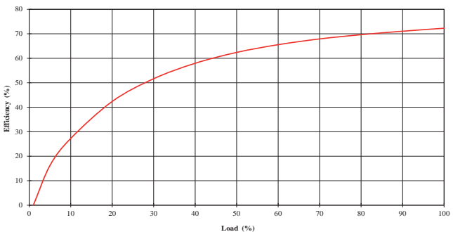
MGJ2D121505MPC
