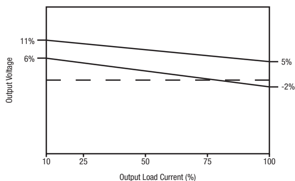
MGJ2D121505MPC
