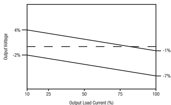
MGJ2D151509MPC
