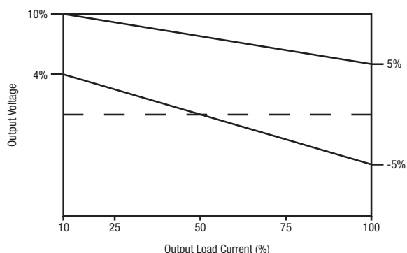
MGJ2D121509MPC
