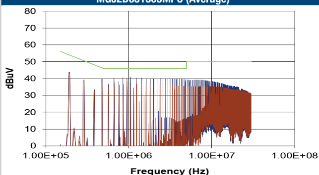
MGJ2D051505MPC (Average)
