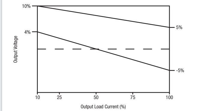
MGJ2D121509MPC
