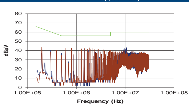
MGJ2D152005MPC (Quasi-Peak)
