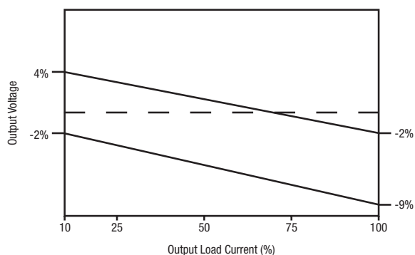
MGJ2D052005MPC
