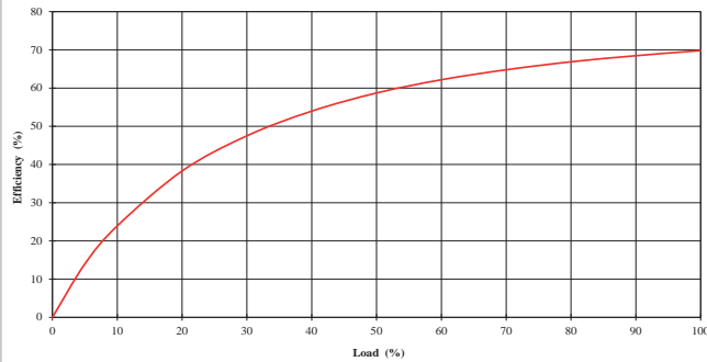
MGJ2D052005MPC
