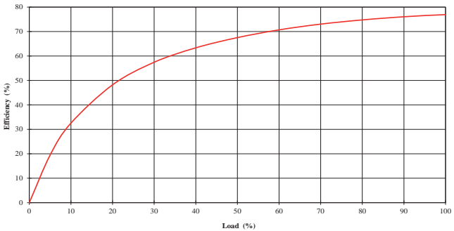
MGJ2D122005MPC
