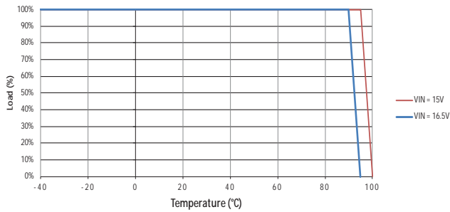
MGJ2D152005MPC
