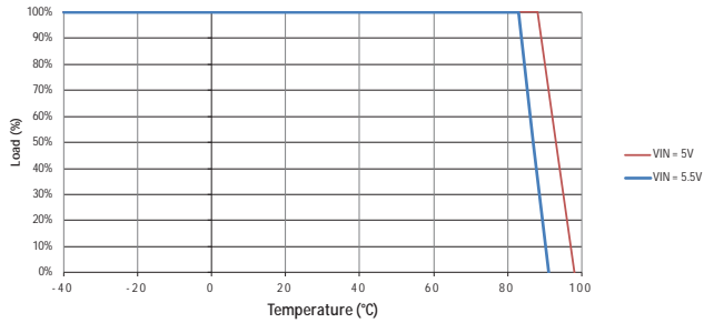
MGJ2D052005MPC
