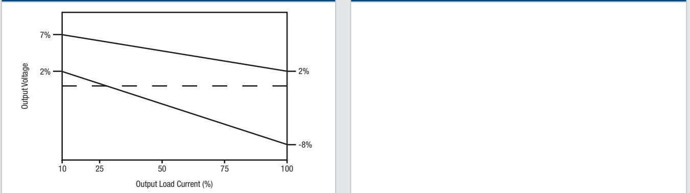
MGJ2D121509MPC
