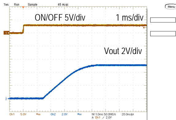
On/Off Enable Delay (Vin=12V, Vout=5.0V, Iout=4A, Cload=400uF)
