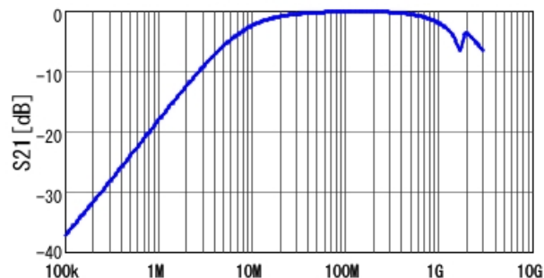
S Parameter S21
